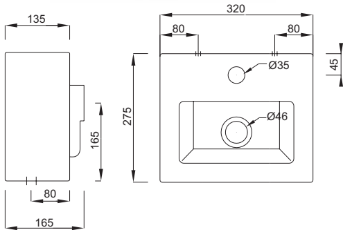
Lavello "FUORI BOX MINI" Basin "FUORI BOX MINI"
