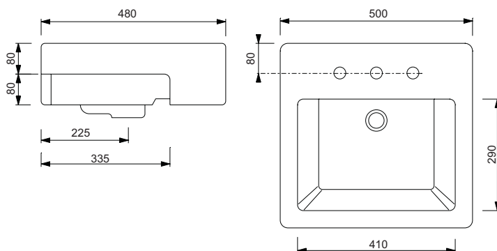
Lavello "FUORI BOX" semincasso Basin "FUORI BOX"
