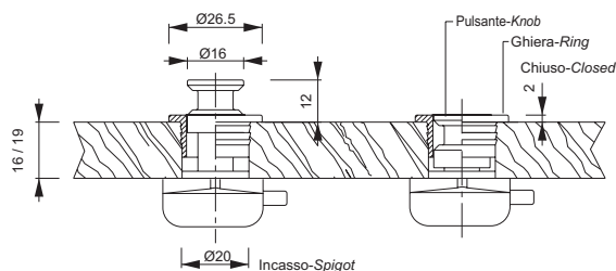
Pulsanti in ottone per portelli e cassetti completo di serratura bianca Brass push lock for cupboard doors with white mechanism
