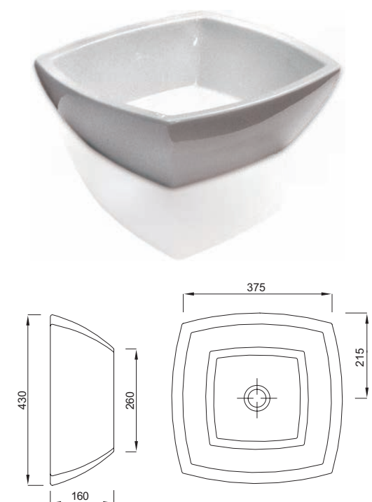
Lavello "FUORI CORNER QUADRO" Basin "FUORI CORNER QUADRO"
