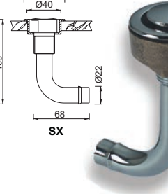
Sinistro 90° - Portagomma Ø22 Left 90° - Hose Ø22
