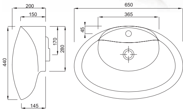
Lavello "FUORI QUOTA" Basin "FUORI QUOTA"
