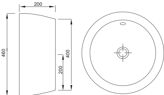
Lavello "FUORI GIRO" Basin "FUORI GIRO"
