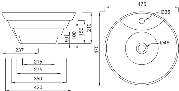
Lavello "FUORI SCALA" Basin "FUORI SCALA"
