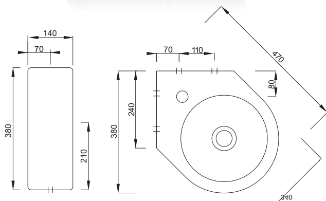
Lavello "MODULA MINI" Basin "MODULA MINI"
