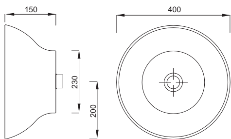
Lavello "FUORI 1" Basin "FUORI 1"
