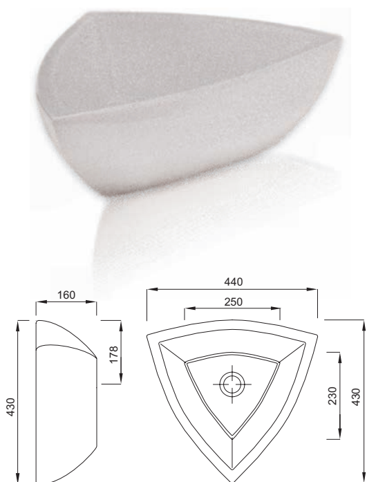
Lavello "FUORI CORNER" Basin "FUORI CORNER"
