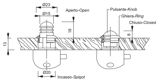
Pulsante in ottone per portelli e cassetti completo di serratura bianca Brass push lock for cupboard doors with white mechanism
