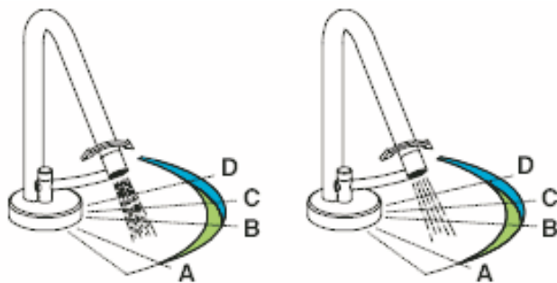
Funzionamento regolatore di portata/Flow regulation working.
