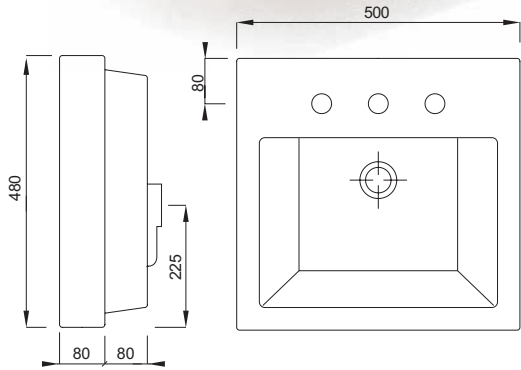
Lavello "FUORI BOX INCASSO" Basin "FUORI BOX INCASSO"
