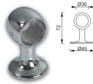
Intermedio con prigioniero M10 Middle with stud fastening M10
