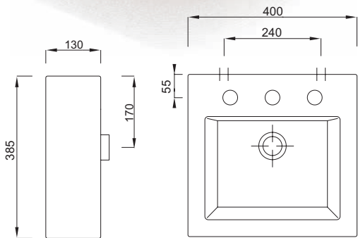
Lavello "FUORI BOX 40" Basin "FUORI BOX 40"
