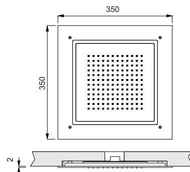
Soffione incasso a filo Shower head recessed fitting
