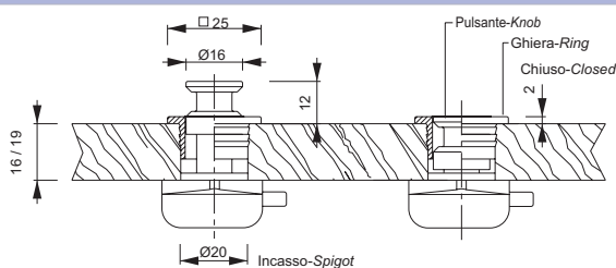
Pulsanti in ottone per portelli e cassetti completo di serratura bianca Brass push lock for cupboard doors with white mechanism
