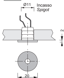
Fissaggio a pressione Pressure fixing
