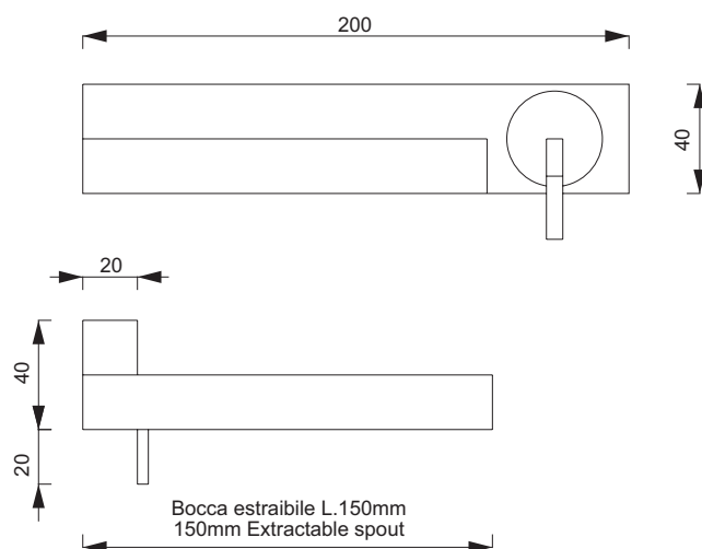
Miscelatore lavabo a parete con bocca estraibile da 150mm Wall flexible basin mixer with 150 mm extractable spout
