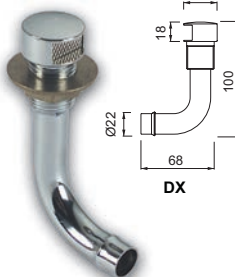
Destro a 90° - Portagomma Ø22 Right 90° - Hose Ø22
