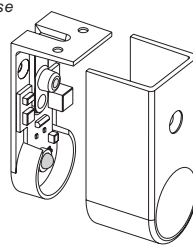
Coperchio estetico Aesthetic cover
