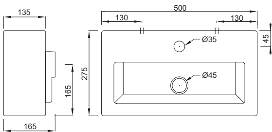
Lavello "FUORI BOX 27" Basin "FUORI BOX 27"
