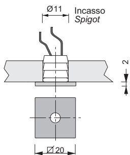
Fissaggio a pressione Pressure fixing
