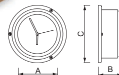
Orologio al quarzo con cassa marina fissa in ottone, indicante il movimento e il senso delle maree attraverso l'uso della quarta lancetta azzurra
